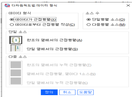
[PROXSCAL 대화상자]
