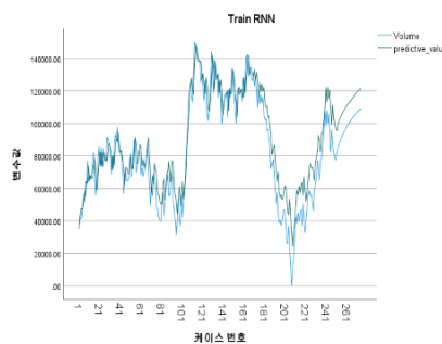
[RNN시계열학습-그래프]
